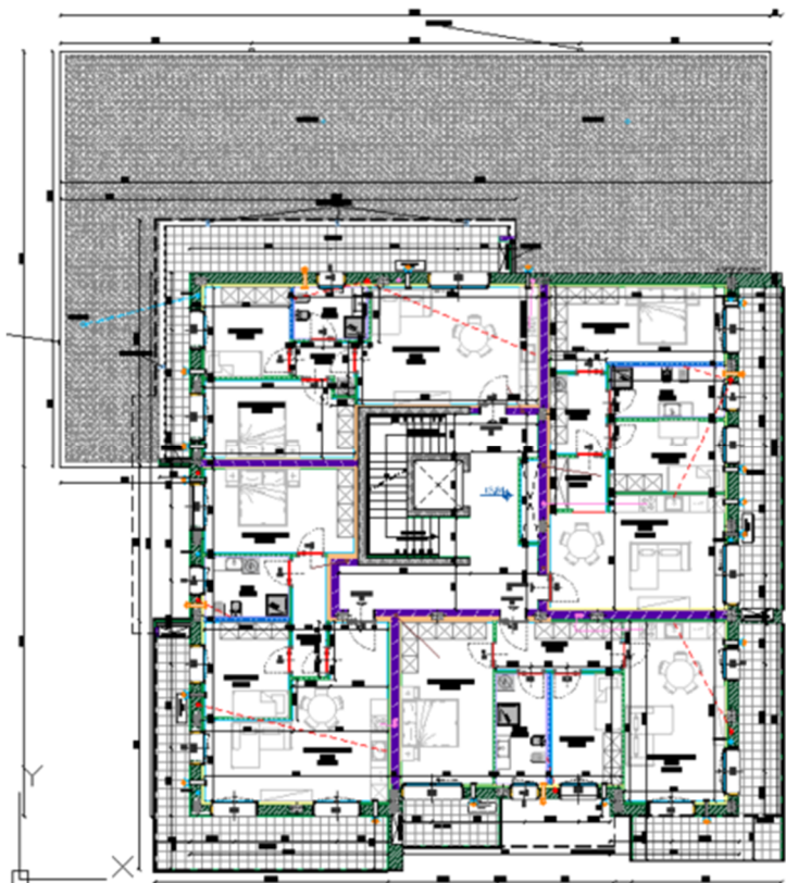
Schema Piano Primo
